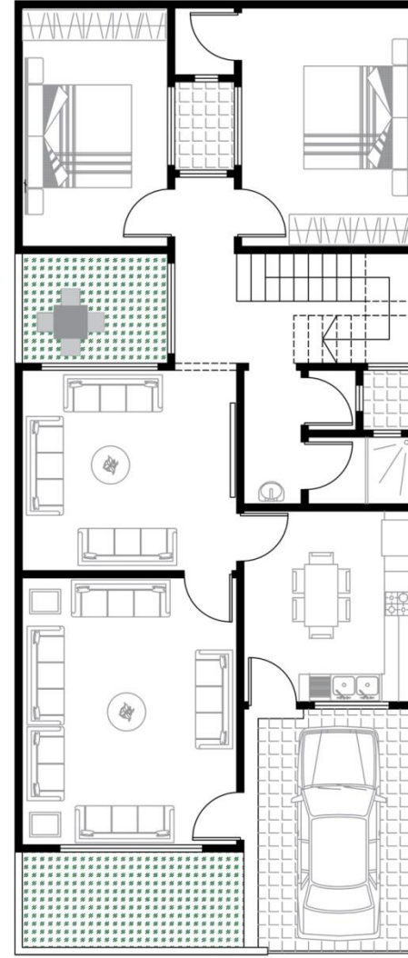
الطابق الارضي
