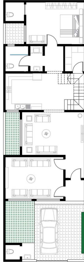
الطابق الارضي
