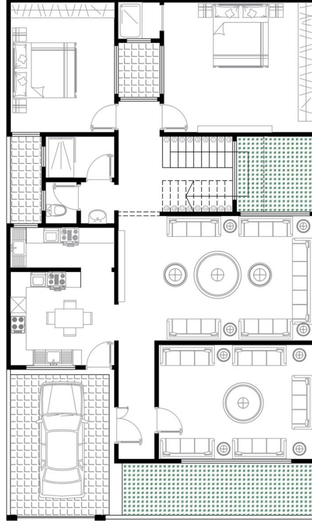
الطابق الارضي
