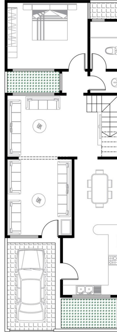
الطابق الارضي
